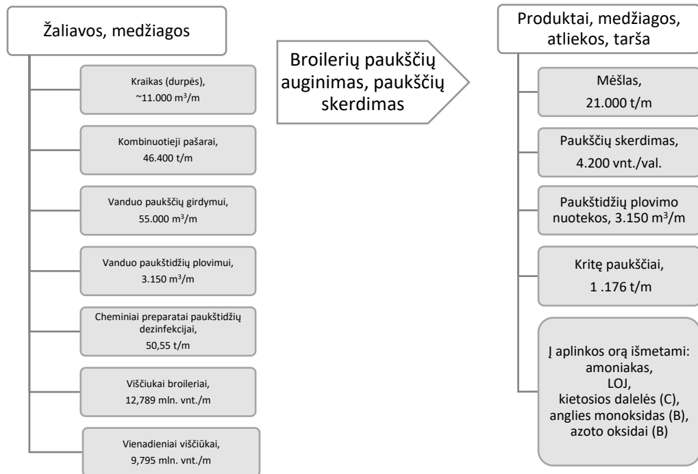
10.1 pav. Broilerių paukščių auginimo supaprastinta procesų schema
